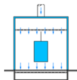
KABINA APLIKACYJNA system dolnego nawiewu
